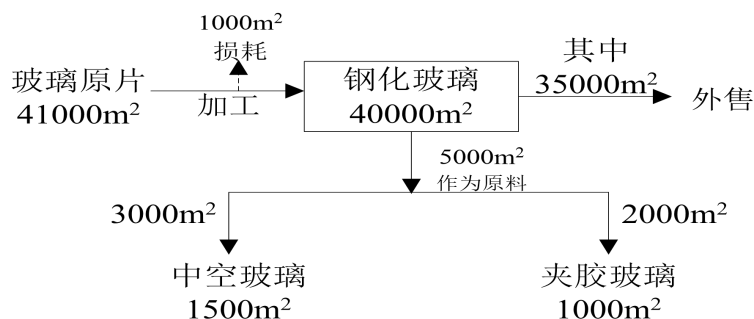
图 2-1 产品流向示意图
