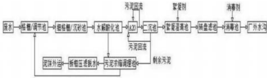
图 4-1 青龙污水处理厂工艺流程图
