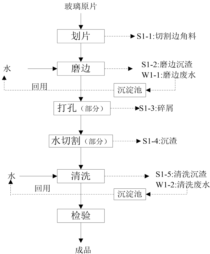
图 2-3 钢化玻璃工艺流程及产污环节图
