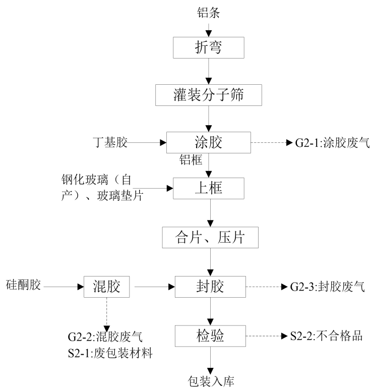
图 2-4 中空玻璃工艺流程及产污环节图
